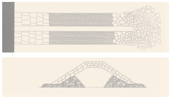
Een bovenaanzicht en een dwarsdoorsnede door een klassiek stortsteenstrandhoofd (VL)
